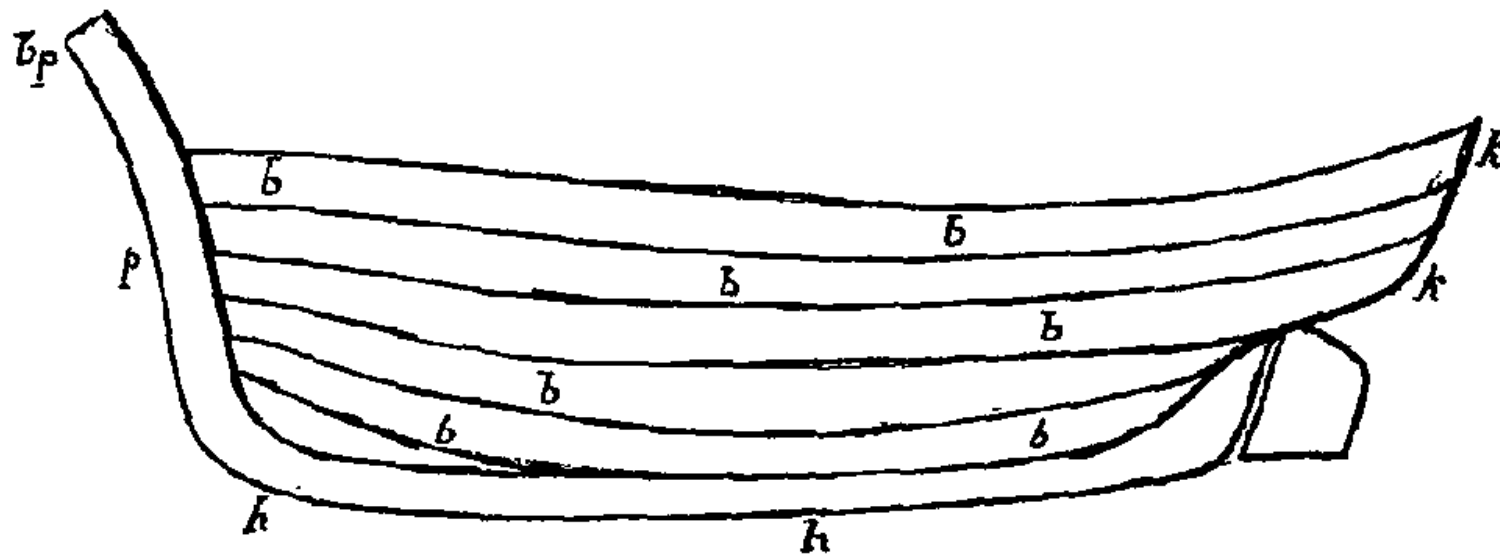
Coque d'une barque de pêche ou de cabotage rifaine, à Tétouan.
