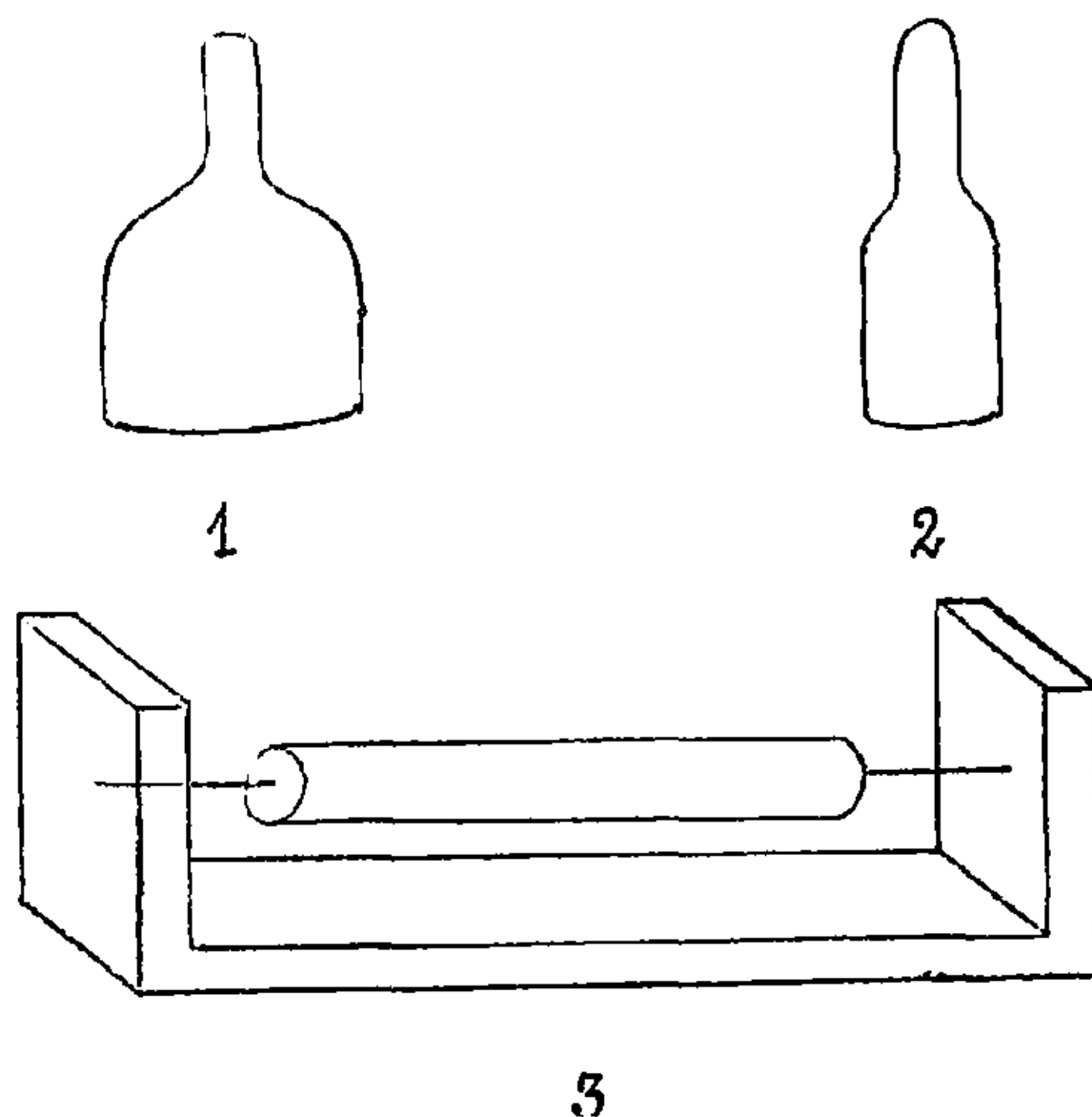
1. Le khefif ; — 2. Le thekil , maillets de cordonniers tétouanais, faits par les tourneurs tétouanais; — 3. Le tour des tourneurs tétouanais.
